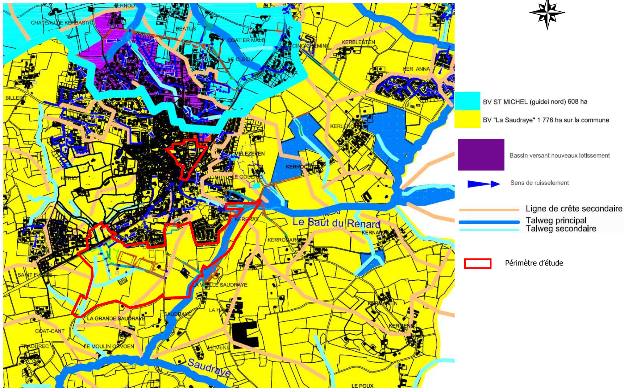
Figure 11 : Fonctionnement hydraulique au droit du site d'étude Source : Schéma directeur des eaux pluviales de la commune de Guidel, Hors échelle
