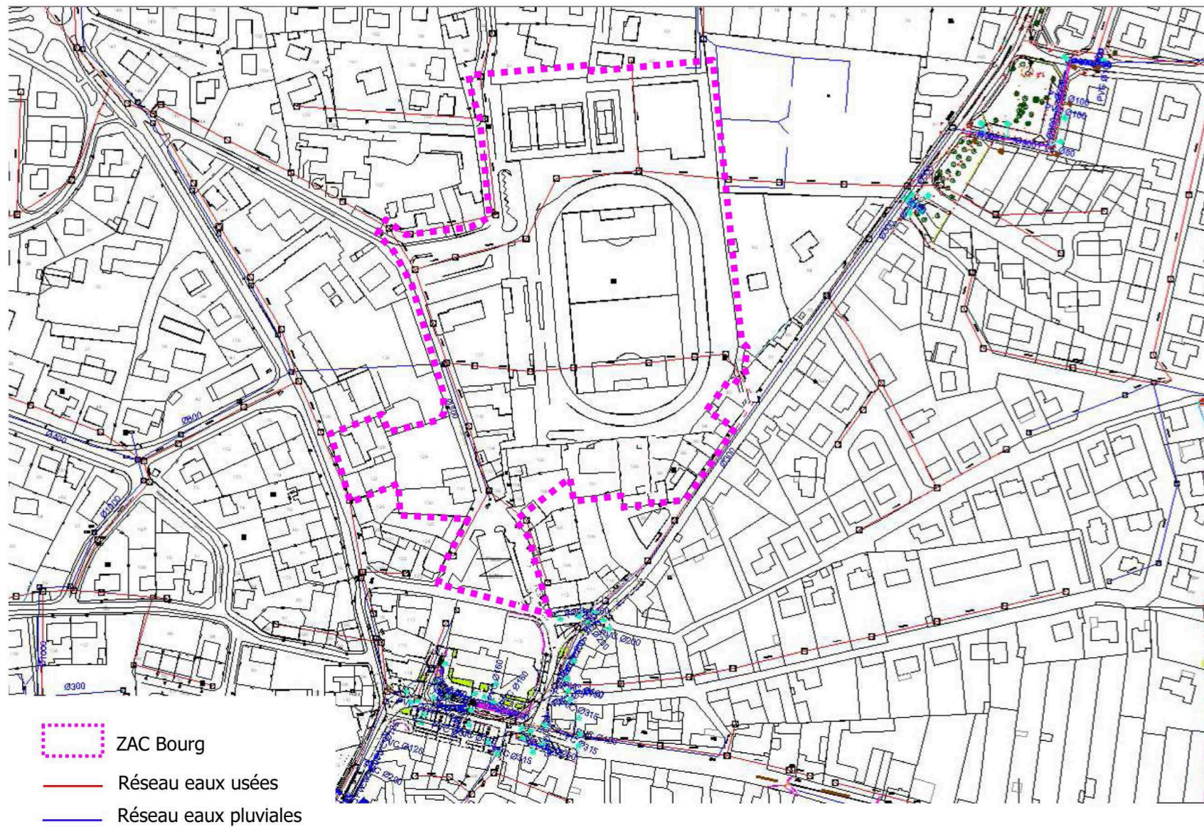
Figure 40 : Réseau eaux usées et eaux pluviales au droit de la ZAC du bourg Hors échelle, Source : PLU de Guidel
