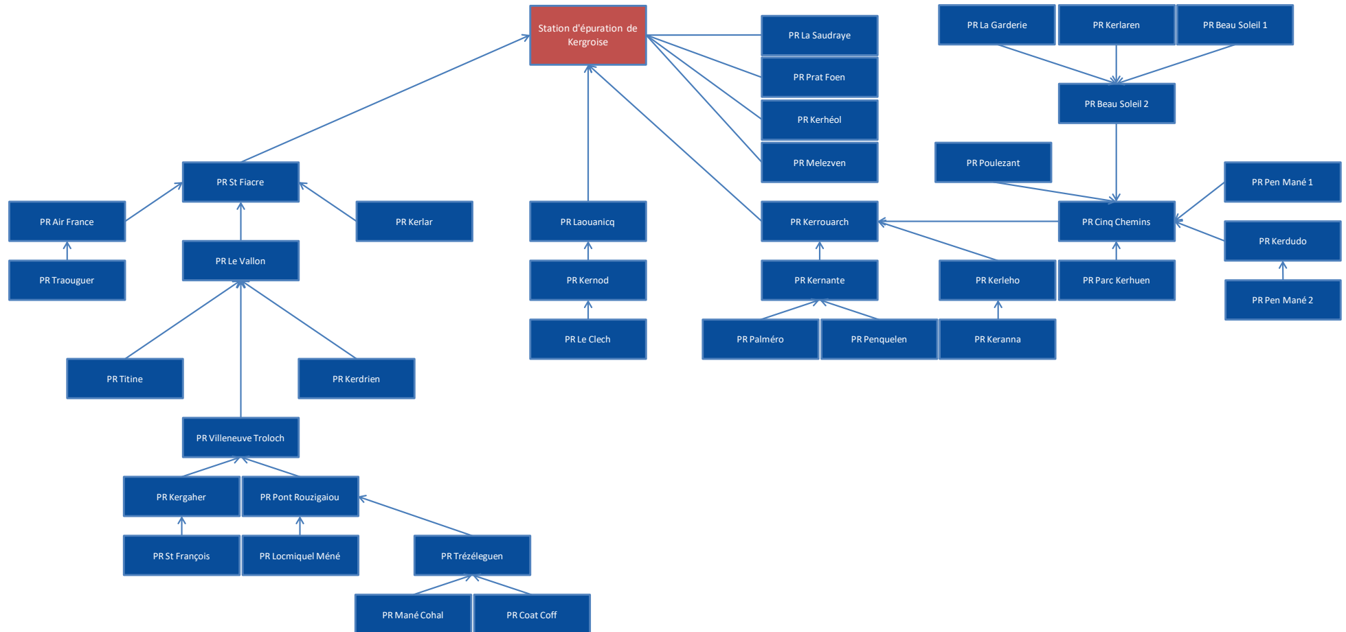
Figure 14 : Synoptique PR – Station d'épuration de Kergroise
